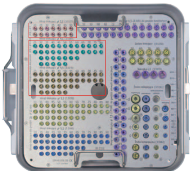
40.5058.200 Behälter für Verriegelungsschrauben für Nägel Charfix2 (Im Container ohne Implantate) Stand for Charfix2 locking elements (set with box without implants) Contenedor para elementos de bloqueo Charfix2 (set con caja sin implantes)
