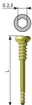
Kompressionsschraube M4 Compression screw M4 Tornillo de compresión M4
